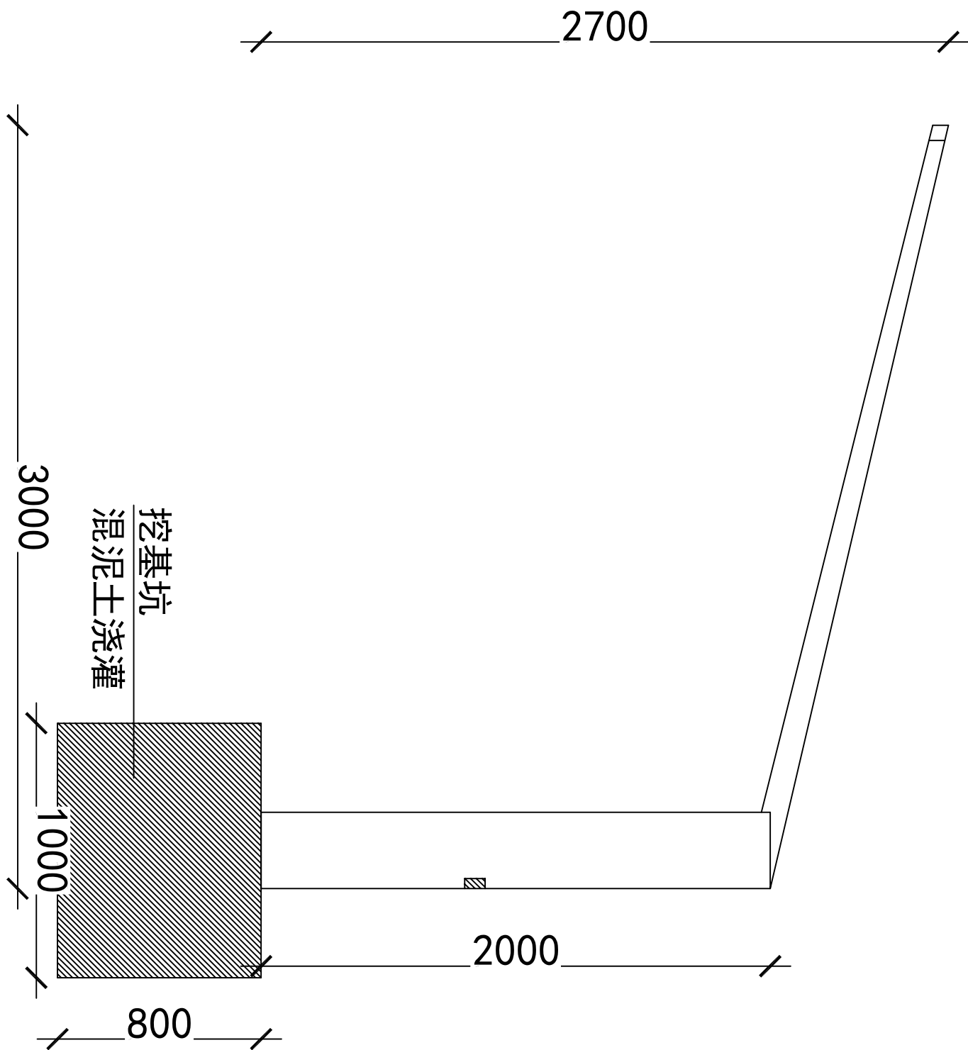
侧视图
